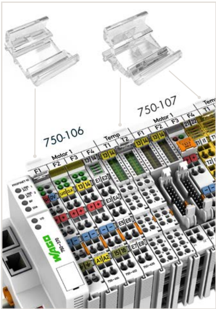
适于标记条(2009-110)或WMB卷装标记牌(2009-115)的组标记支架
